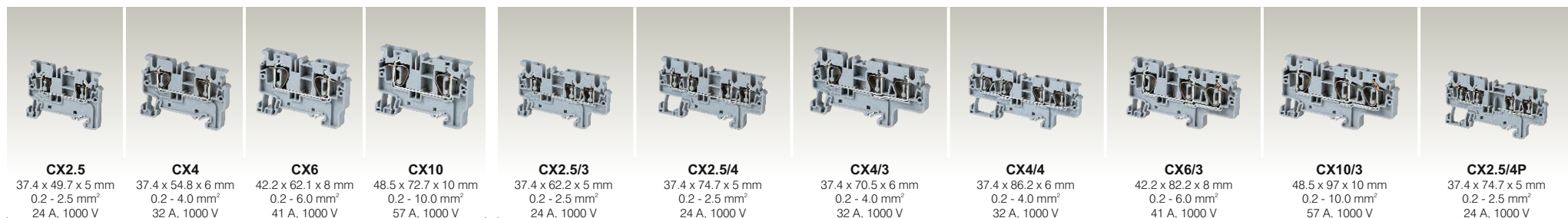
Clemas para alimentaci3n
